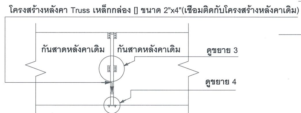
แบบขยาย 2 มาตรฐาน NO SCALE
